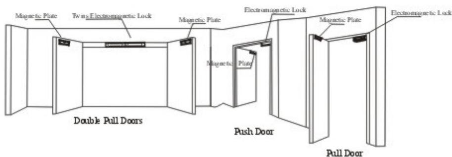
Pull Door
